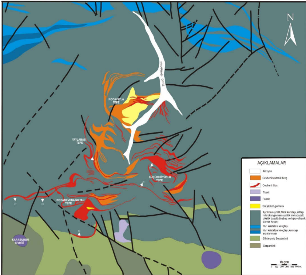
Sivrihisar- Beylikova - Okcu Köyü - Kızılcaören Toryum (Basnasit-Barit-Florit Kompleks Cevher) Yatağı
