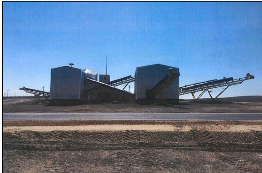
Keskin inşaat ve yıkıntı atıkları geri kazanım tesisi konkasörü (sabit kırıcı)
