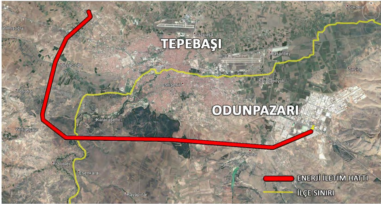
Şekil 3. 154 KV Eskişehir 3 – Eskişehir 2 Enerji İletim Hattı
