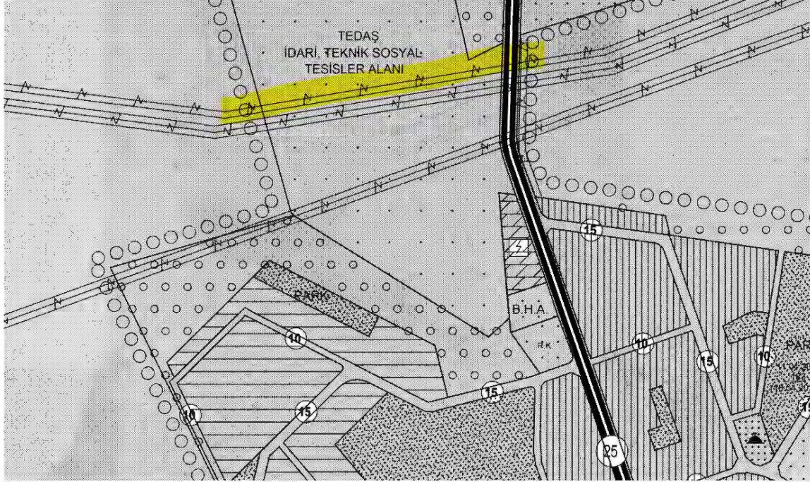
Şekil 6. 1/5000 Ölçekli Nazım İmar Planı, Pafta 17P
