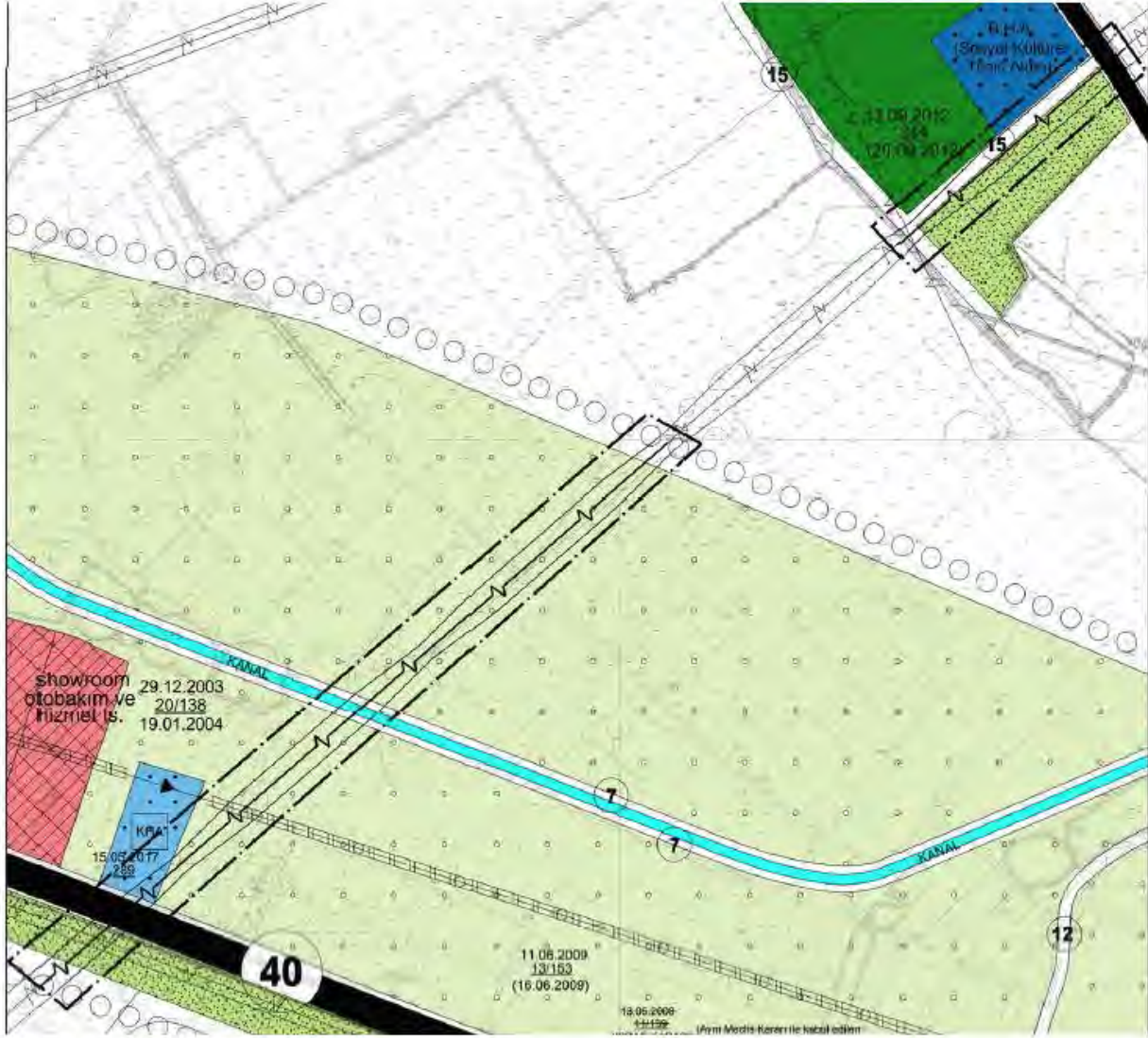
Şekil 14. 1/5000 Ölçekli Nazım İmar Planı Değişikliği Teklifi, Pafta 22K
